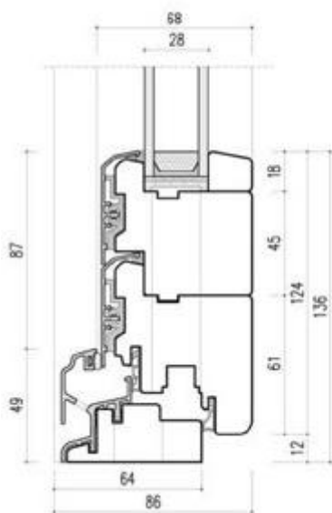
Sezione Verticale Balcone
