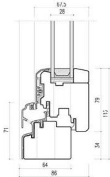
Sezione Verticale Finestra
