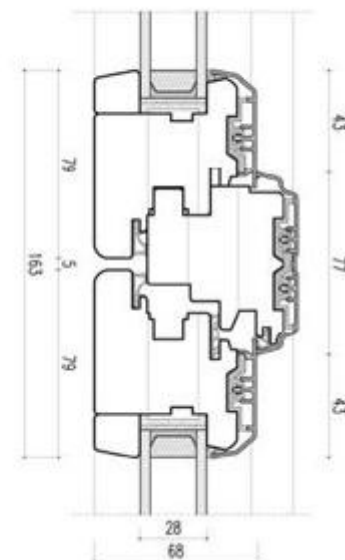
Montante mobile Finestra e Balcone
