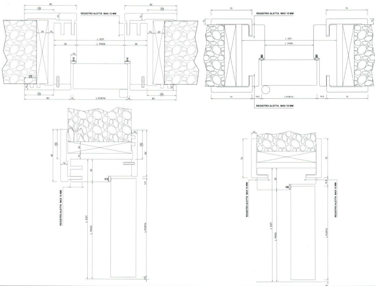
DETTAGLI TECNICI: COLLEZIONE OLIMPO (cassa linea e cassa standard)
